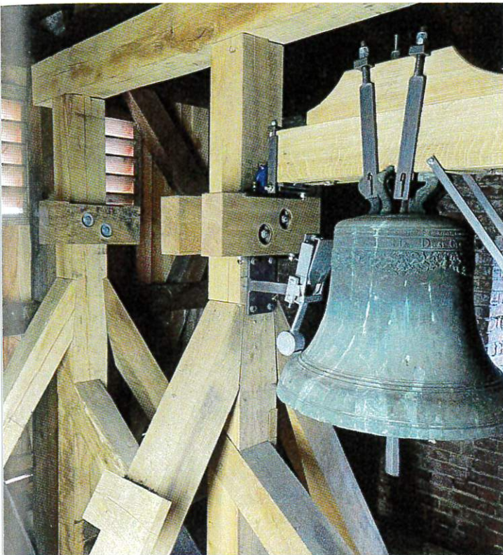
Der neue Glockenstuhl mit einem Platz für die zweite Glocke
